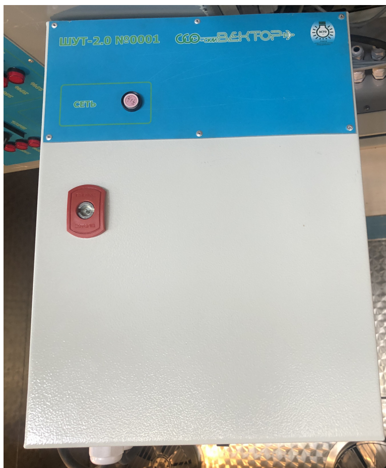
Регулирующий трансформатор (ШУТ-2.0)
